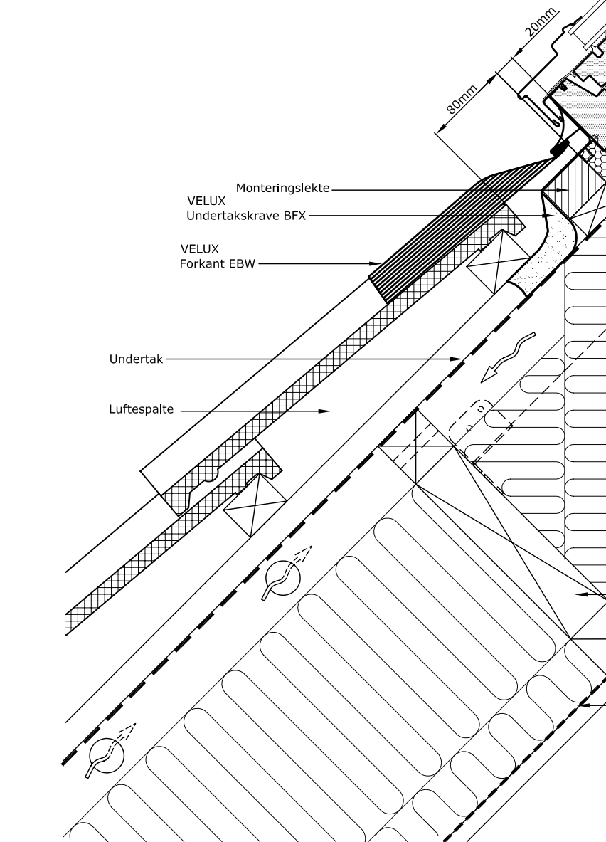
Skisse vinkelrett på tak 1:20
