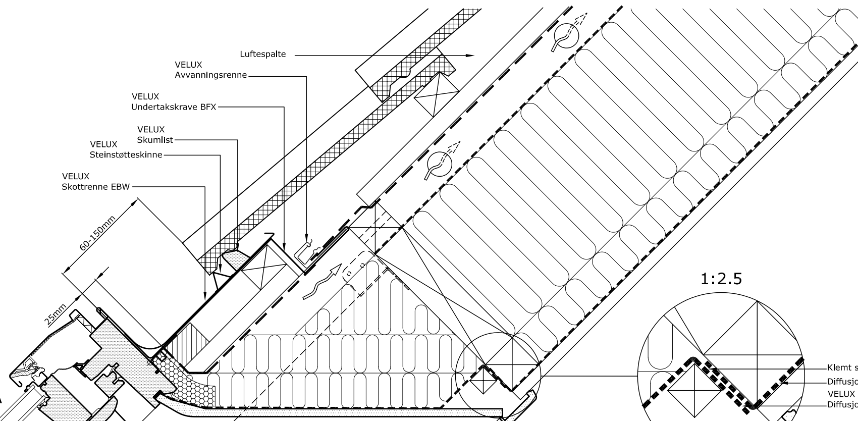
Snitt A-A 1:5
