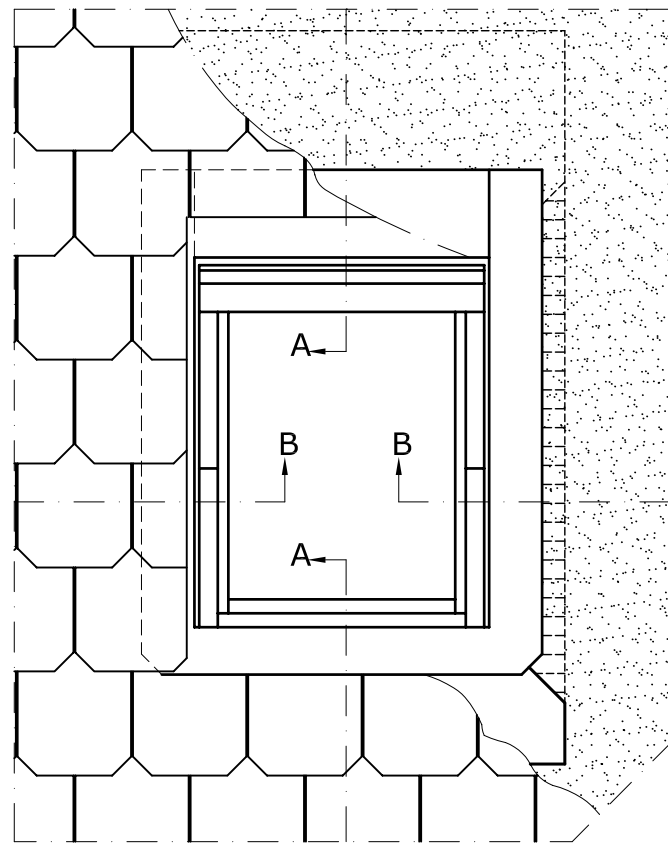
Skisse vinkelrett på tak 1:20
