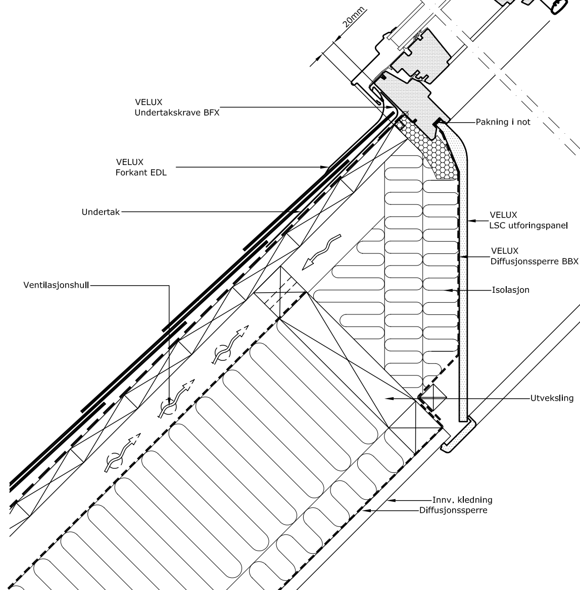
Skisse vinkelrett på tak 1:20
