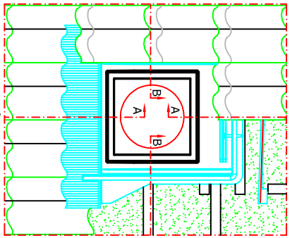
Opstalt vinkelret på tag 1:20
