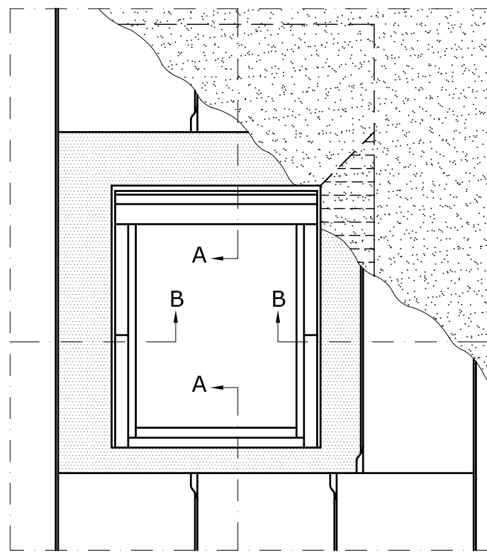
Skisse vinkelrett på tak 1:20
